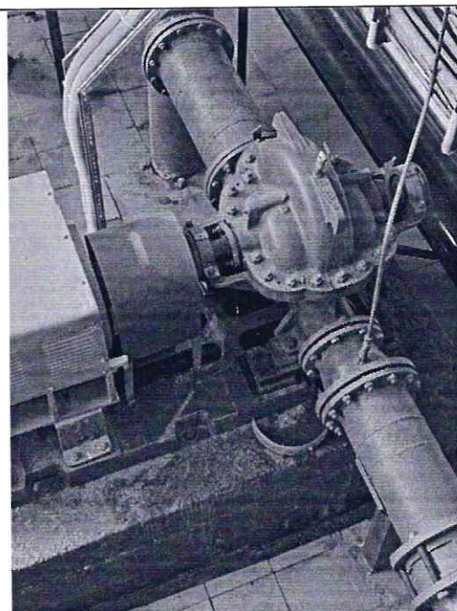
Рис.31. Течь в сальниковом уплотнении вала насоса в насосном зале ВОС
