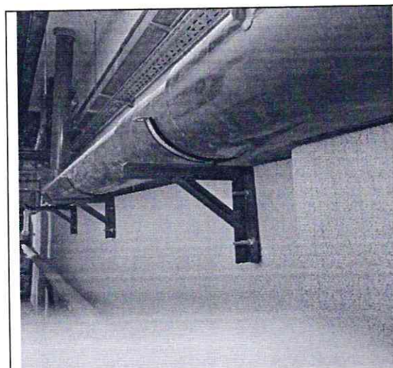
Рис.12. Не закреплены хомуты в отдельных местах
