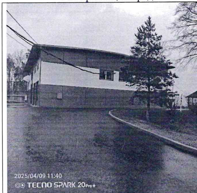
Рис. 24 Общий вид капитального ремонта фасада
