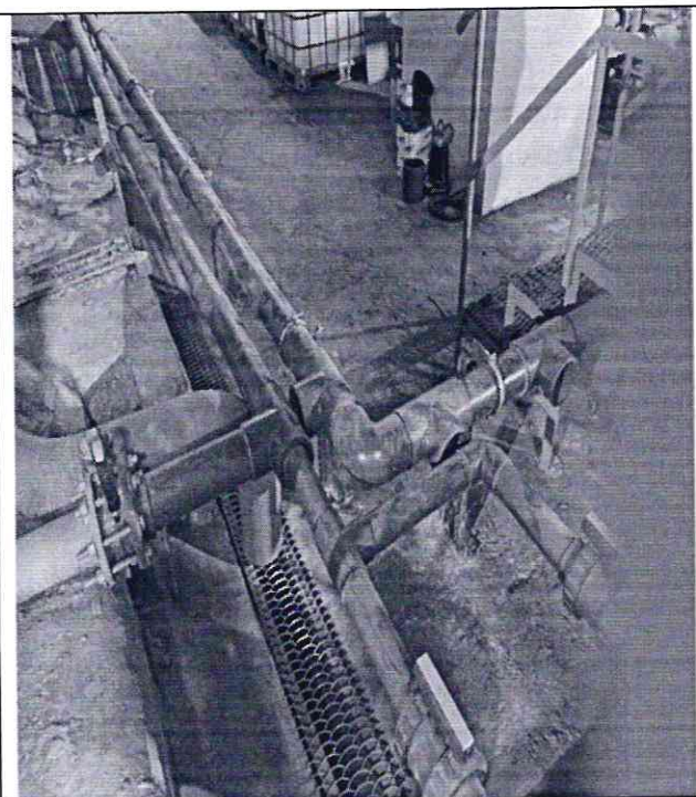
Рис.5. Не связаны трубопроводы
